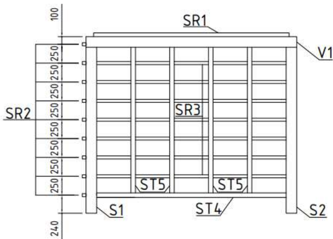
PREDNÝ POHĽAD
