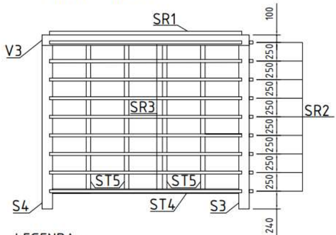
ZADNÝ POHĽAD
